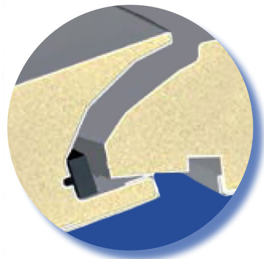
Detalle de la junta
