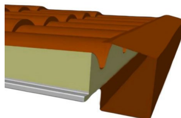
REMATE CANALÓN CERRADO
