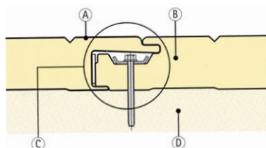
Sistema de tornillo Oculto
