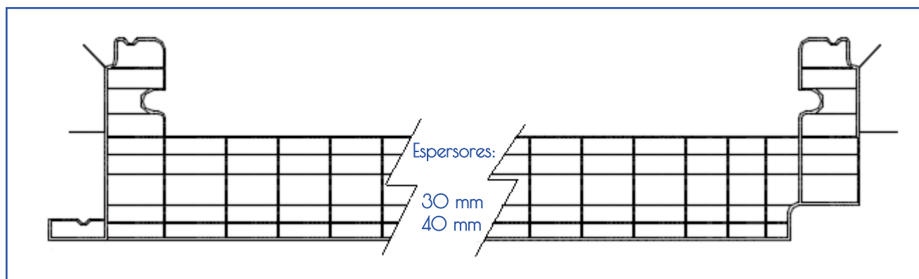
Policarbonato Trapezoidal
