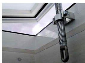
Detalle husillo claraboya
