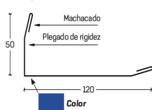
Perfil tipo L50x120 Exterior
